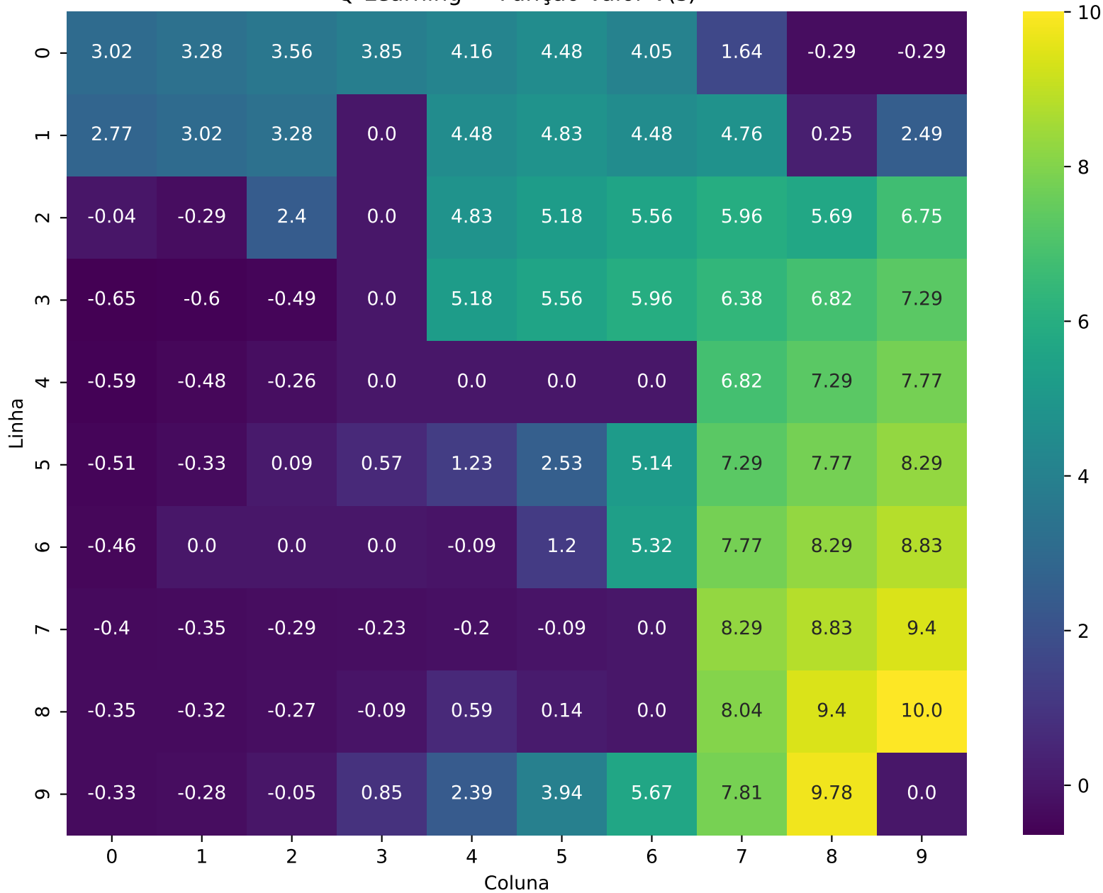
Q-Learning — Função Valor V(s)
